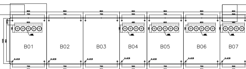
2#配电室平面布置图
