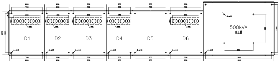
操作面 开关站平面布置图
