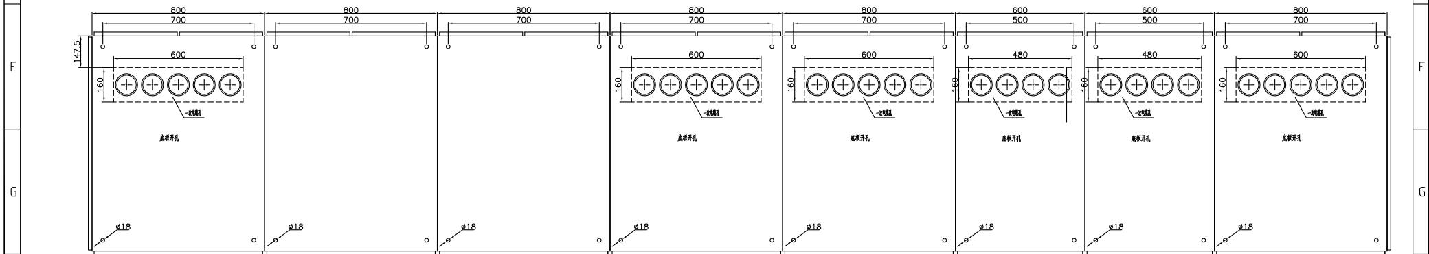
操作面 FOUNDATION DETAIL 基础图
