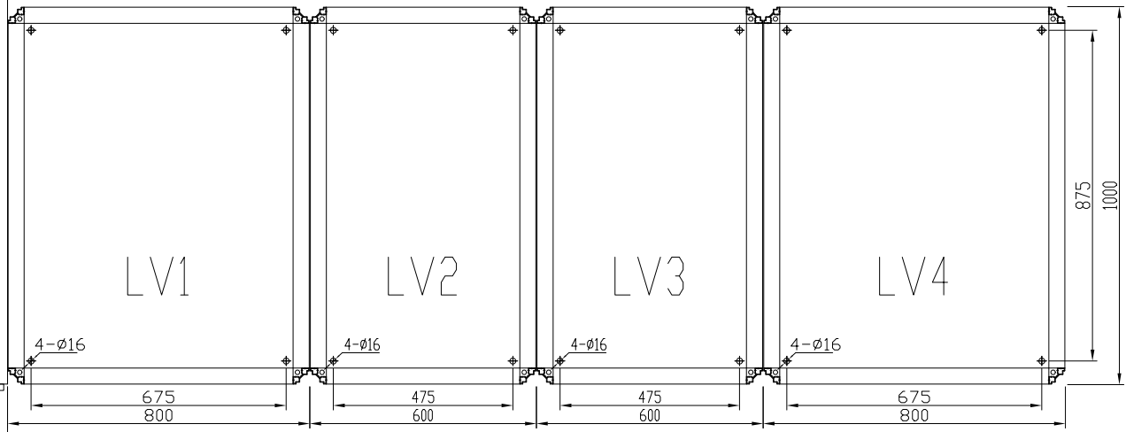
操作面 FOUNDATION DETAIL 基础图
